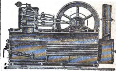
Фиг. 3. Небольшой Л. системы компаунда (вертикальный разрѣзъ)
